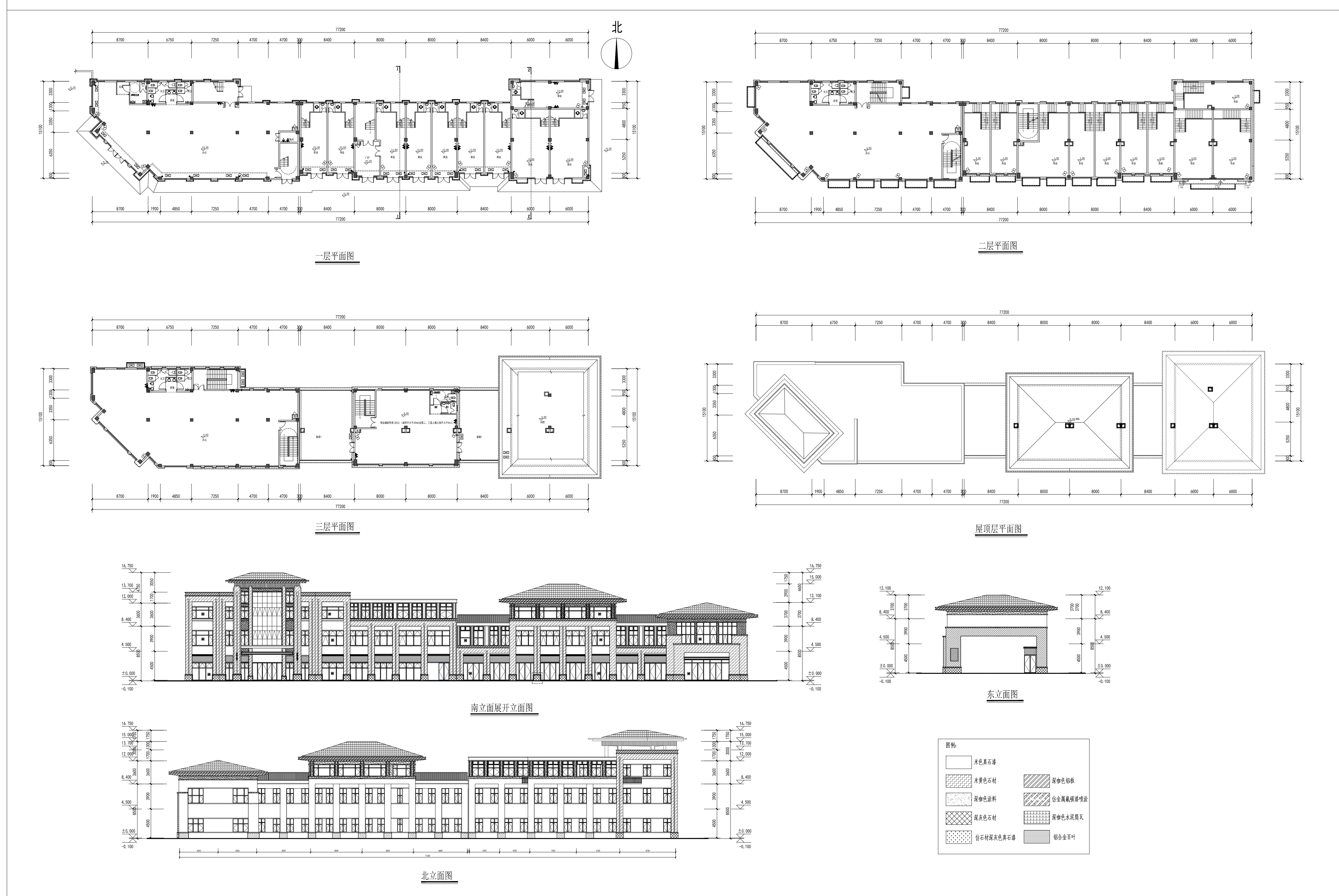
S1#楼调整后平立面图
