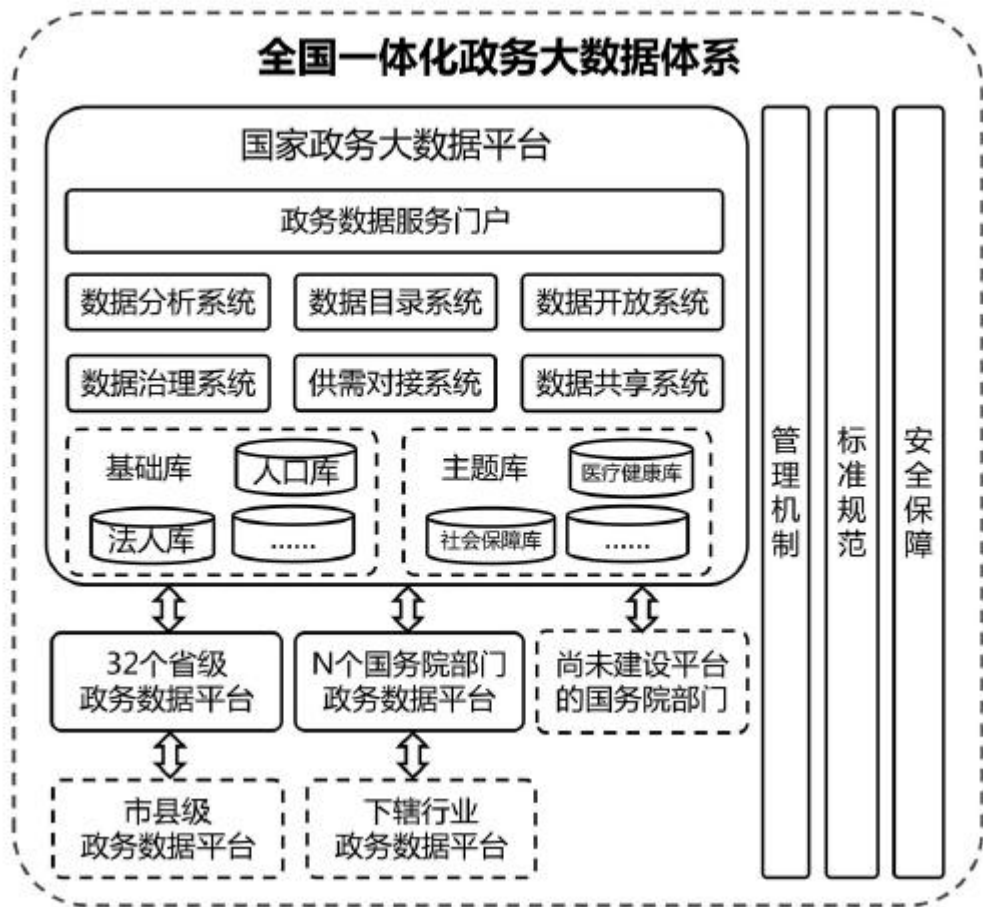
图 1 全国一体化政务大数据体系总体架构图
